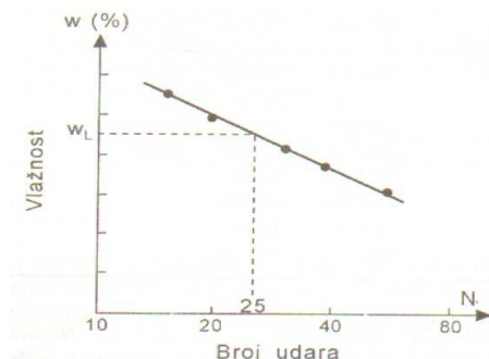
Slika 2.2 Odeđivanje granice tečenja
